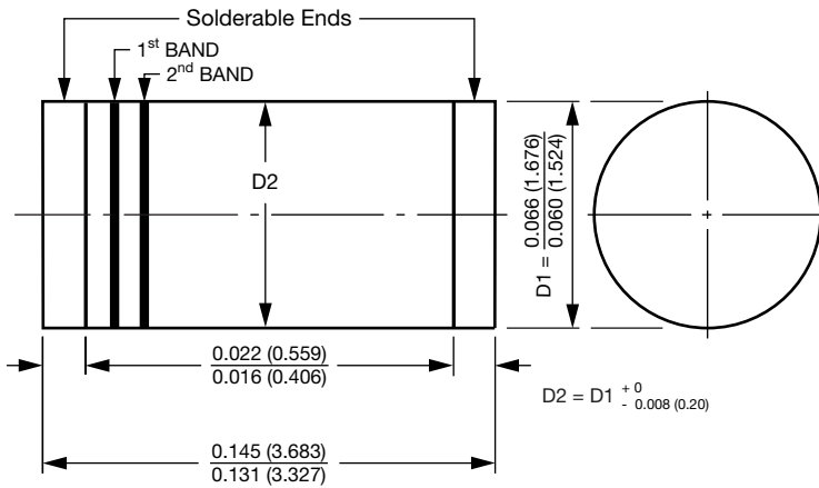
GL34 (DO-213AA)
