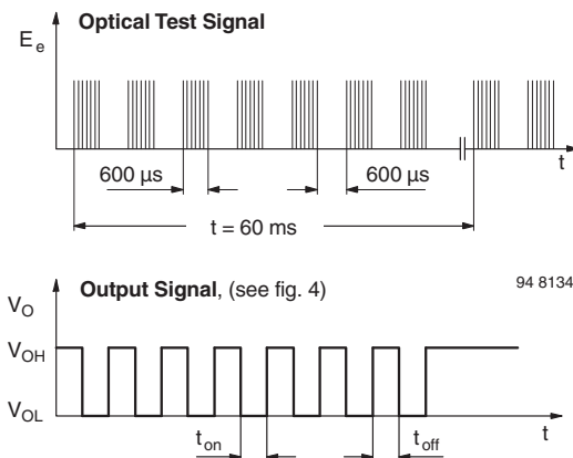
Fig. 1 - Output Function
