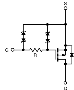
P-Channel MOSFET
