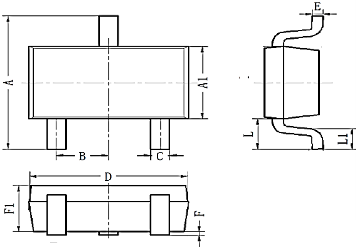
SOT 23-3
