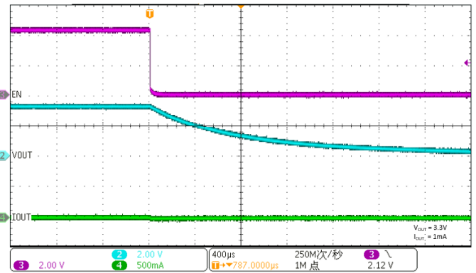
EN Shutdown
