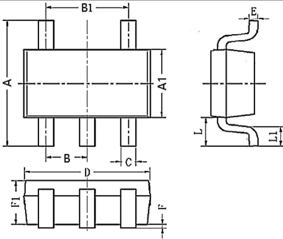
SOT 23-5
