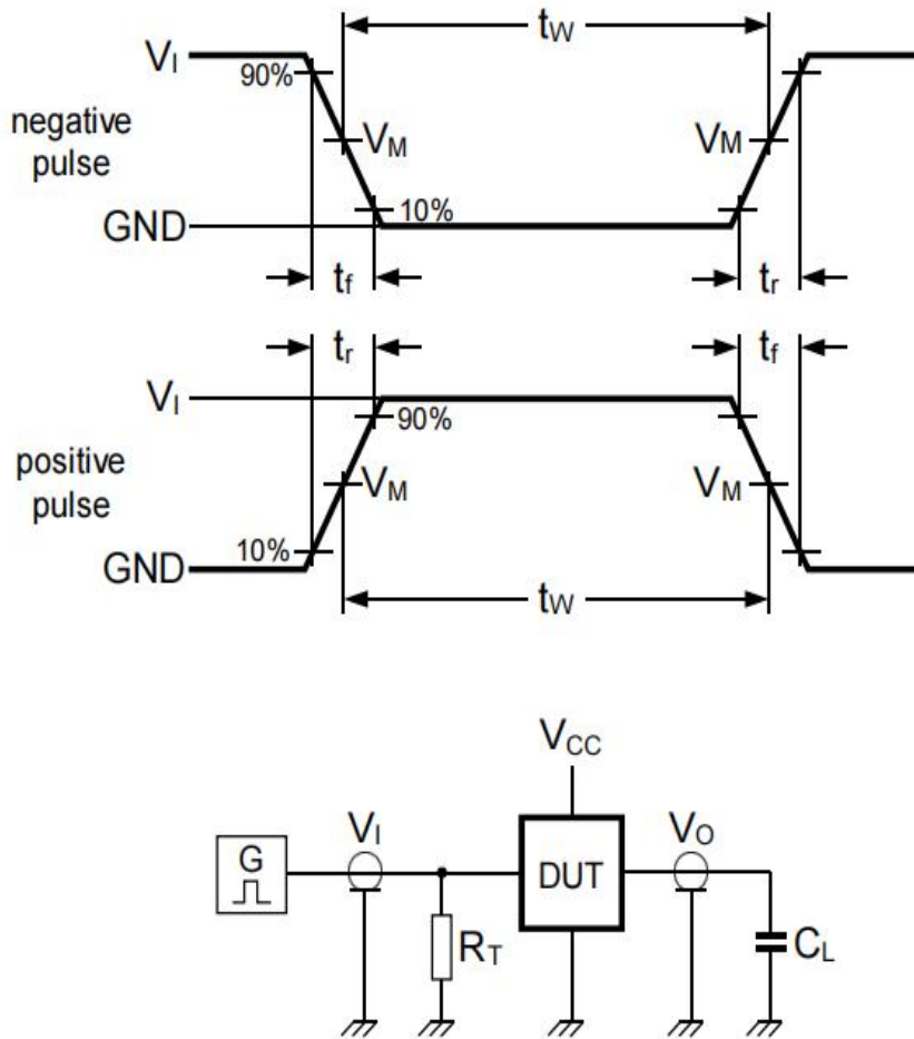
图4 测量开关时间的测试电路
