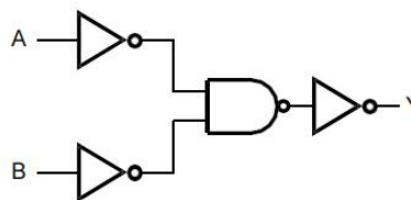
图 3 逻辑框图
