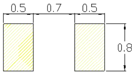
建议焊盘尺寸
