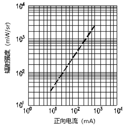
图四：相对强度和正向电流关系曲线
