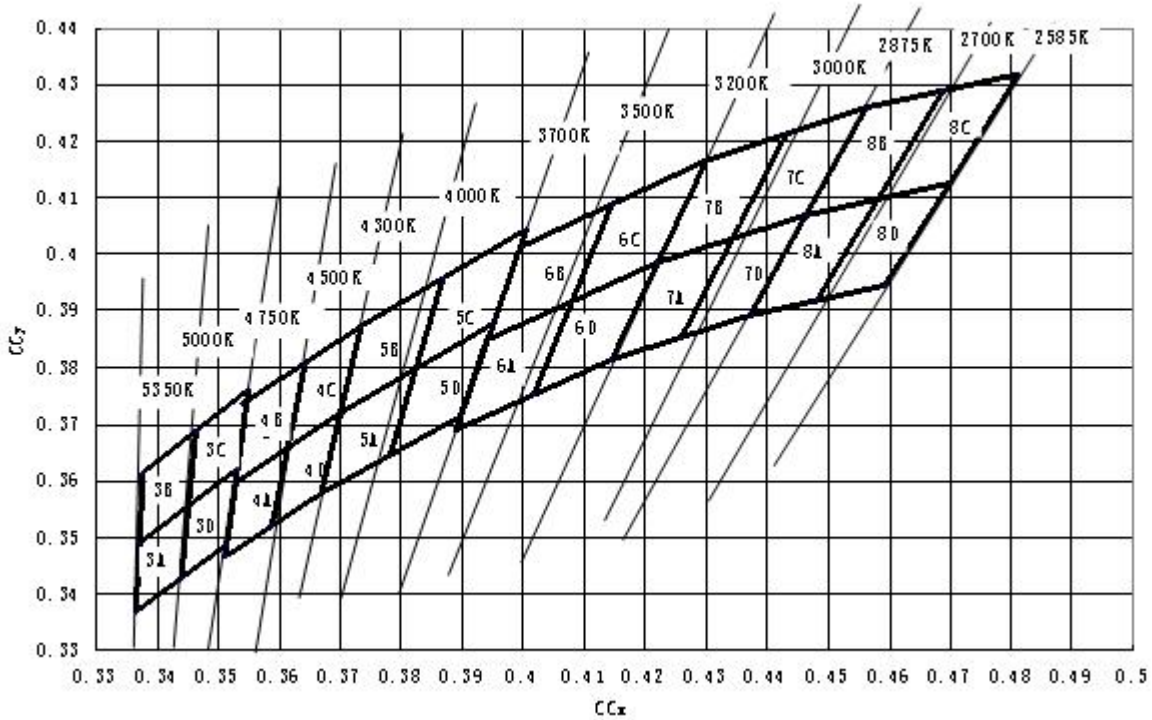
暖白标准色度区域
