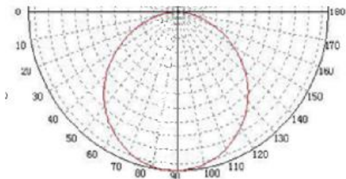
角度-光强 极坐标分布图
