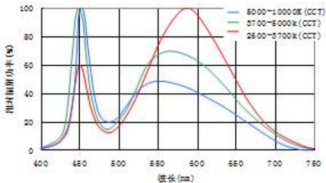
相对光谱功率分布
