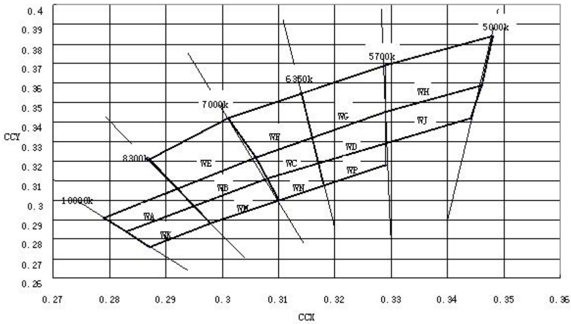
白光标准色度区域
