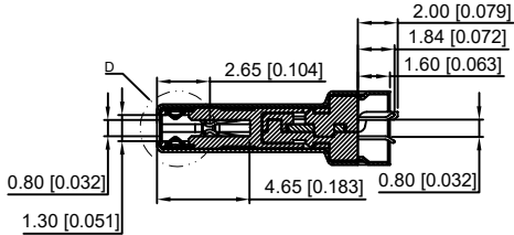
SECT A-A
