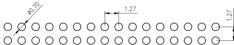
P.C.B LAYOUT
