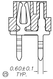
SECTION A-A
