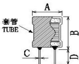
正视图 FRONT VIEW
