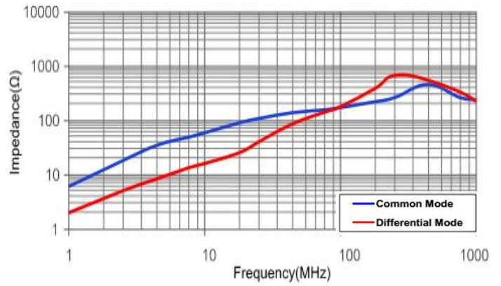
XRACM4520F-151
