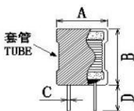
正视图 FRONT VIEW
