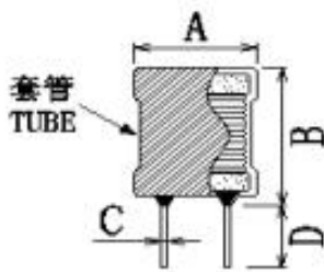
正视图 FRONT VIEW
