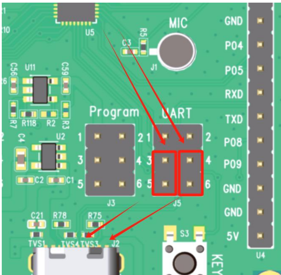
图 8：E3220 开发板 USB 接口选择
