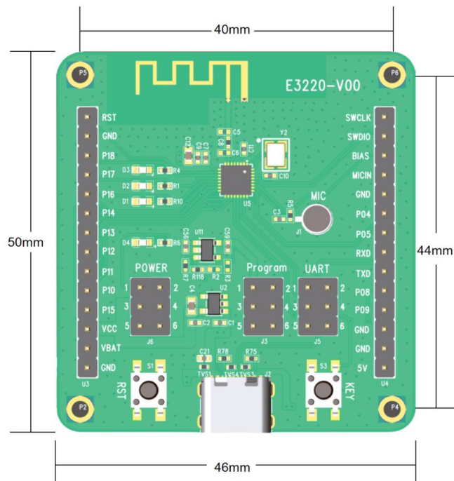
图 2: E3220 开发板尺寸图
