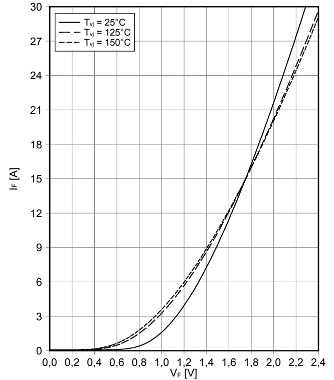
正向偏压特性 二极管, 制动-斩波器 (典型) forward characteristic of Diode, Brake-Chopper (typical)
