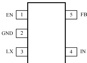
(SOT23-5, TSOT23-5)
