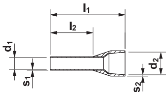
Bild 1 Abmessungen (Toleranzen nach DIN 46228-4)
