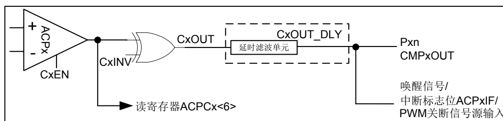
图 6-30 比较器 ACPx 中断产生示意图
