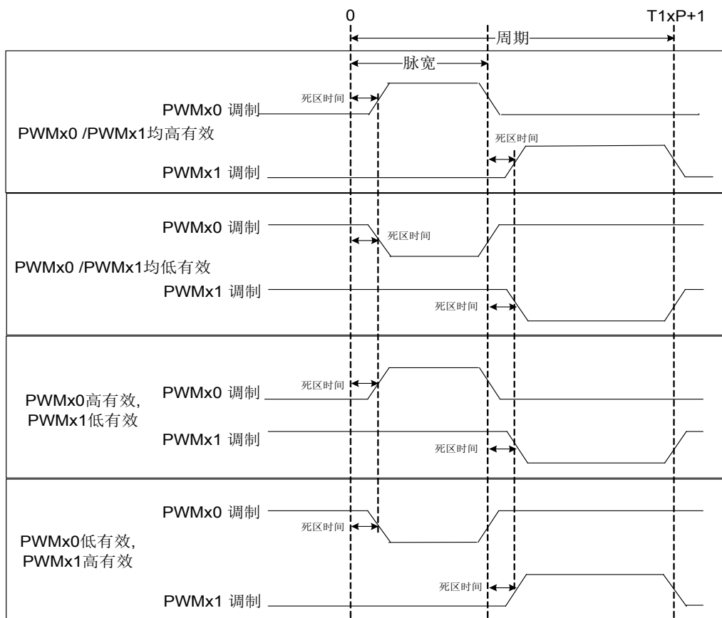
图 6-12 PWM 带死区互补输出极性示意图
