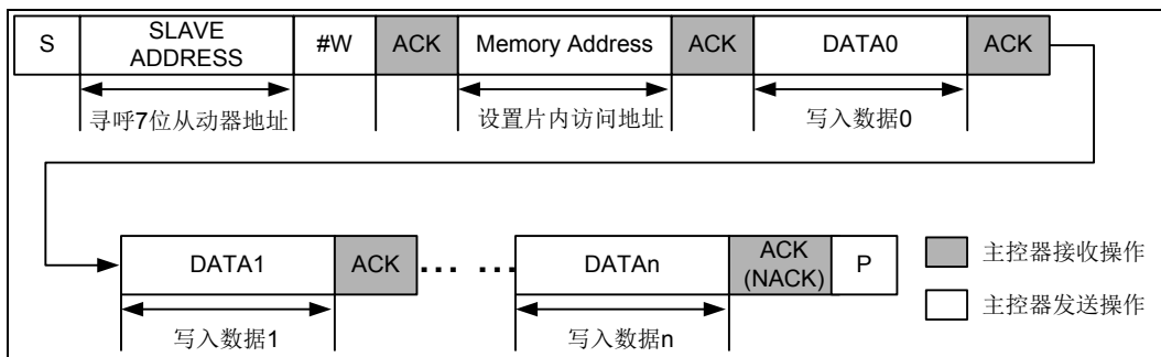
图 6-27 主控器写入从动器数据示意图
