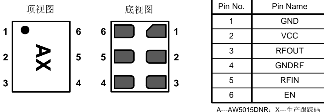
图 1. AW5015 引脚分布及标识图
