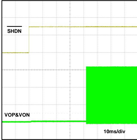
启动时序
