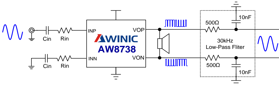
图 6 AW8738 测试电路图
