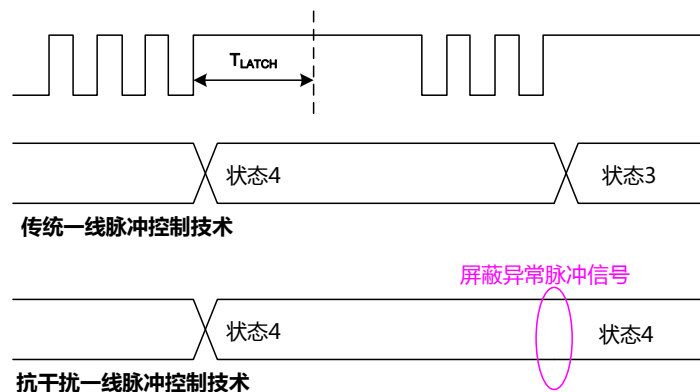
图 15 抗干扰一线脉冲功能示意图
