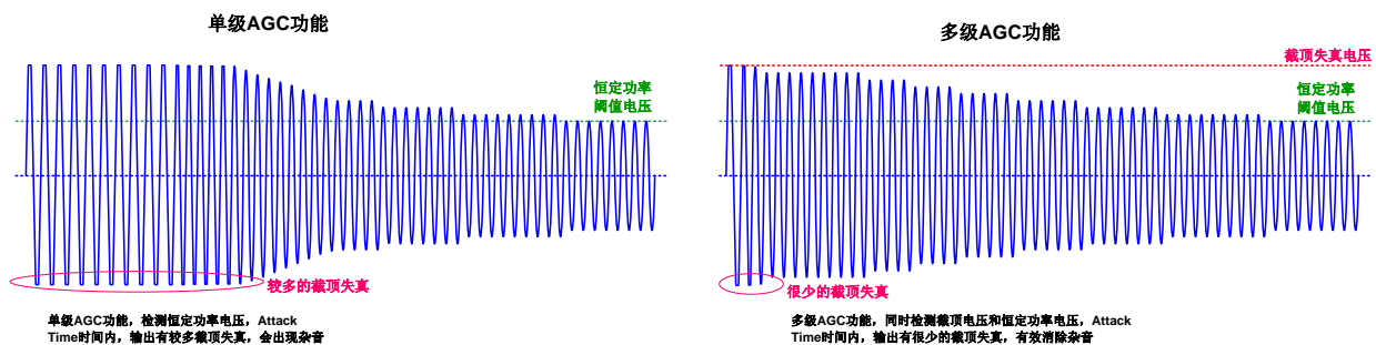
图 10 单级 AGC/多级 AGC 工作原理图
