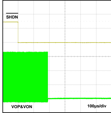
关断时序
