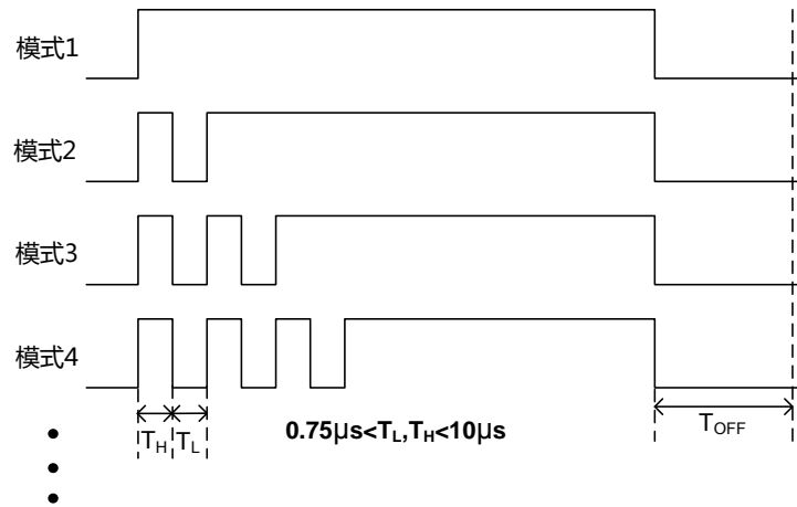
图 16 一线脉冲控制方法
