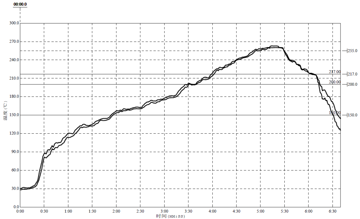
图 10 回流焊曲线图
