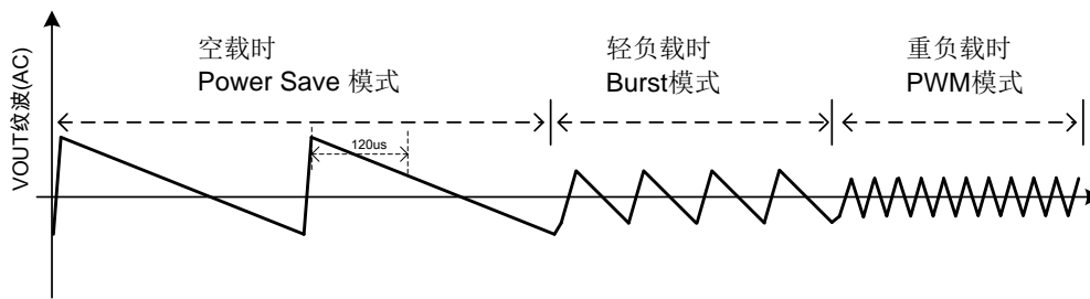
图 4 VOUT 输出纹波示意图
