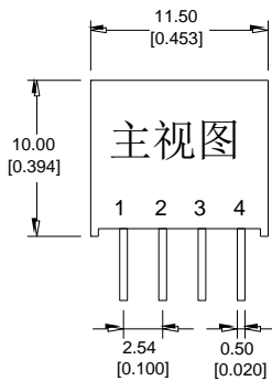
封装尺寸图
