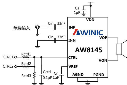
图 3 AW8145 单端输入方式应用图
