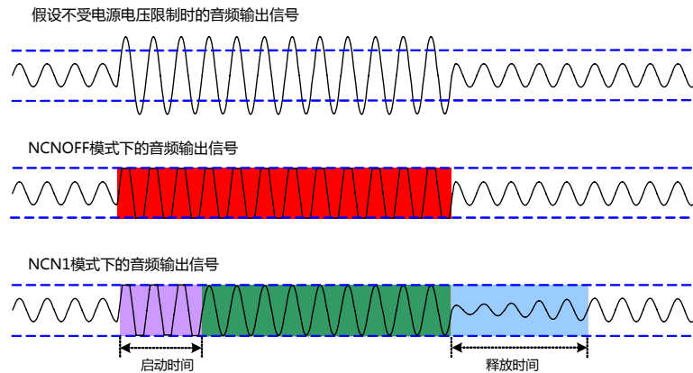
图 6 NCN 功能示意图
