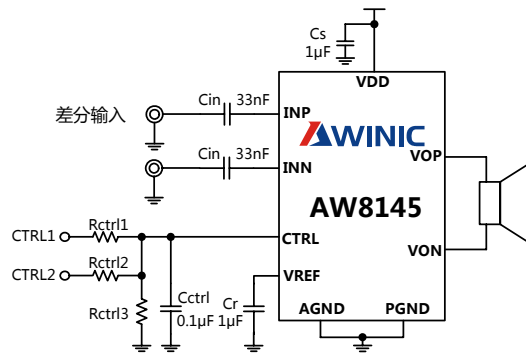
图 2 AW8145 差分输入方式应用图
