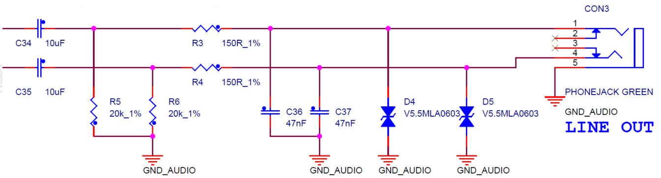
图 7 LINE OUT
