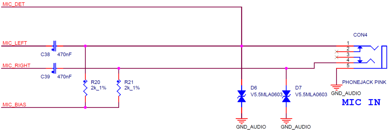
图 8 MIC IN
