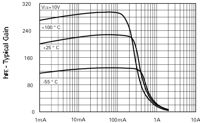
h_{FE} \text{ v } I_C
