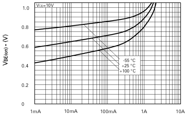
V_{BE(on)} \text{ v } I_C
