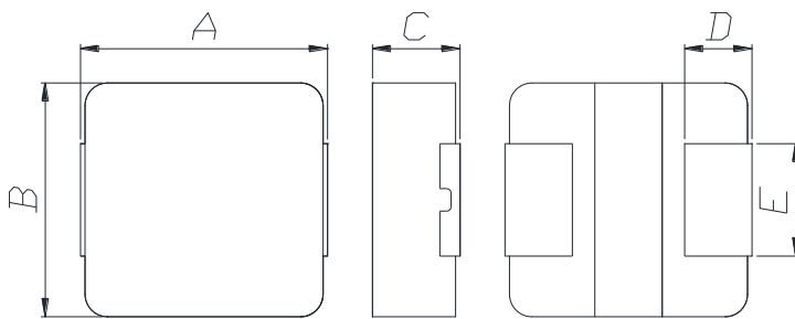
Dimension (Unit:mm)
