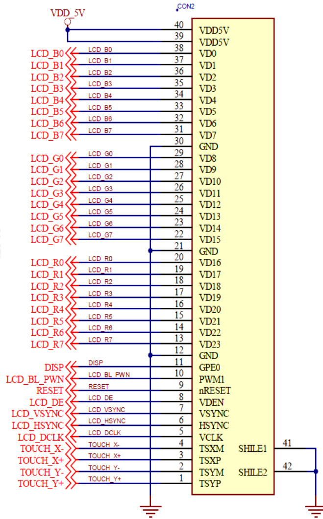
图 6 CON2 接口引脚定义
