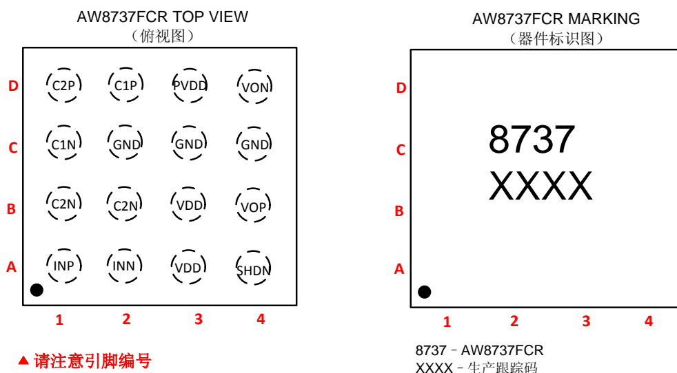
图 2 AW8737FCR 引脚分布俯视图及器件标识图
