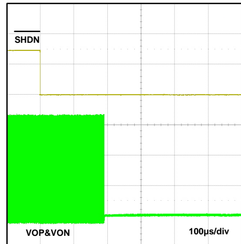
关断时序
