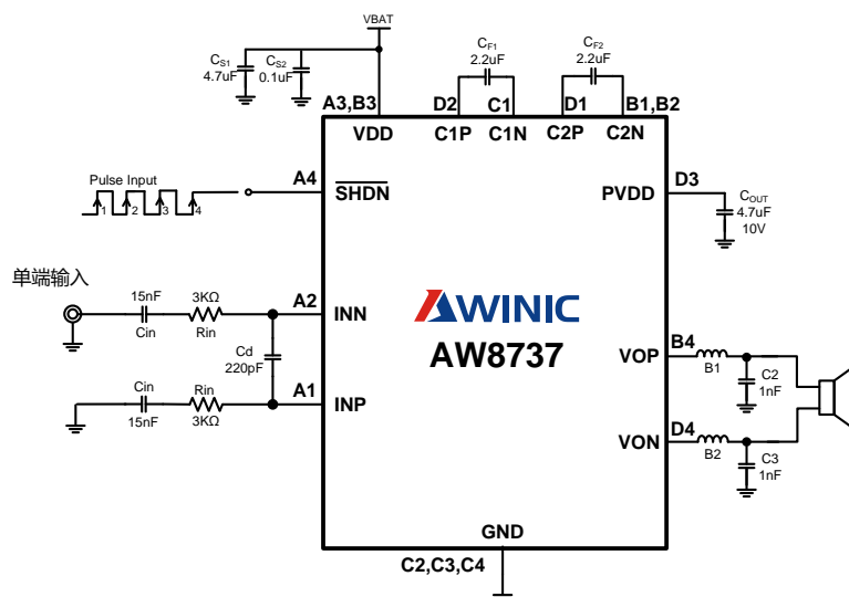
图 1 AW8737 单端输入方式应用图
