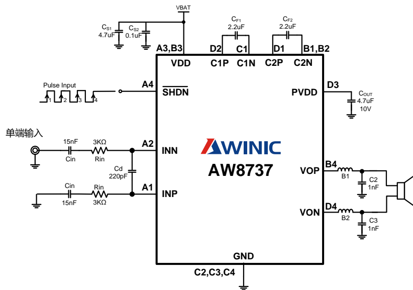
图 4 AW8737 单端输入方式应用图 (注1)
