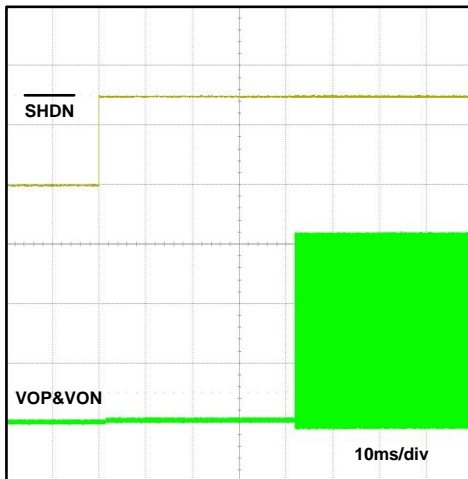
启动时序
