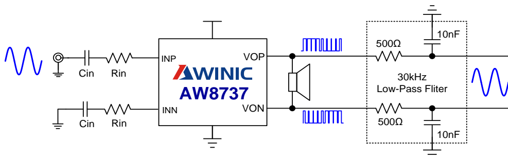
图 6 AW8737 测试电路图
