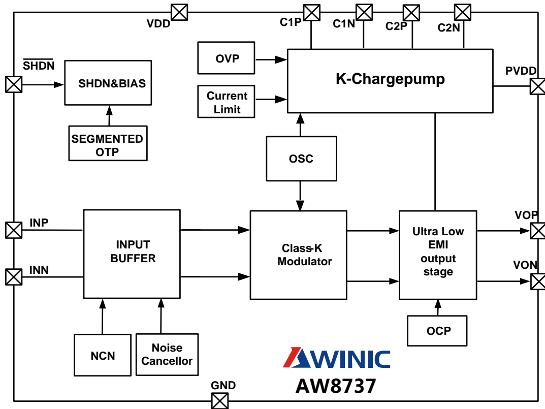
图 3 AW8737 功能框图
