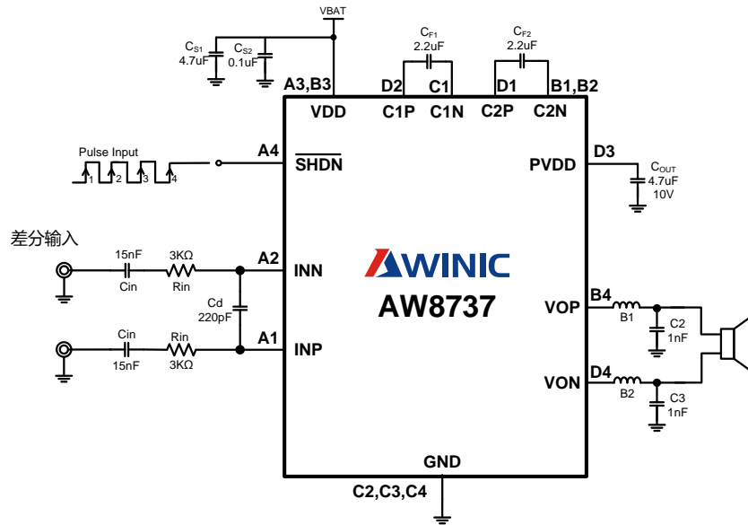
图 5 AW8737 差分输入方式应用图
