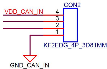
图 6 CON2 连接器 (CAN0 接口)
