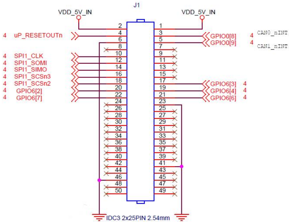
图 5 J1 连接器引脚定义
