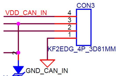
图 7 CON3 连接器 (CAN1 接口)
