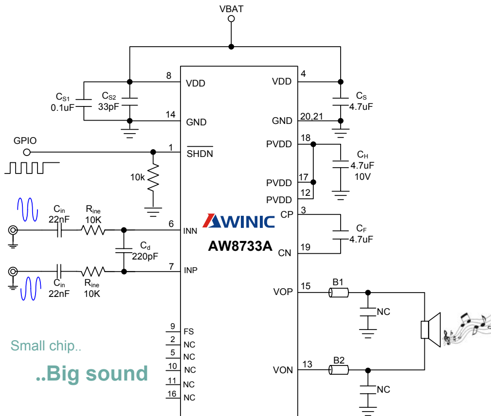
图3 AW8733A 差分输入方式典型应用图（注2）
