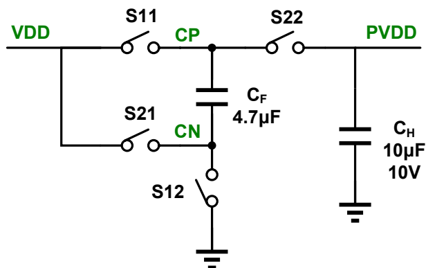
图 12 电荷泵原理图
