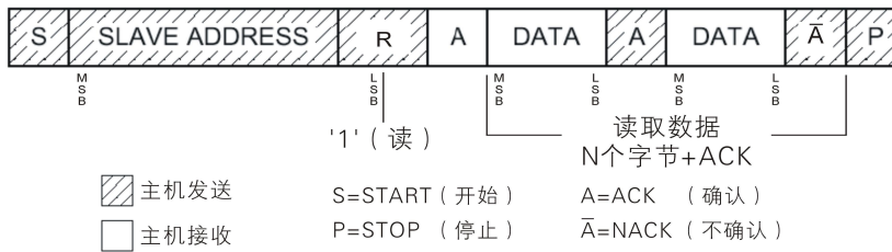
图 12: I 2 C 总线主机从从机接收数据的基本格式
