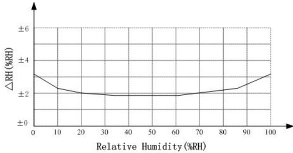
图 2: 25°C 时 AM2322 的相对湿度最大误差
