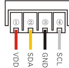
图 4: AM2322 接线图
