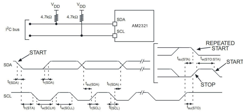
图 13: AM2322 典型的 I2C 总线应用电路和时序图
