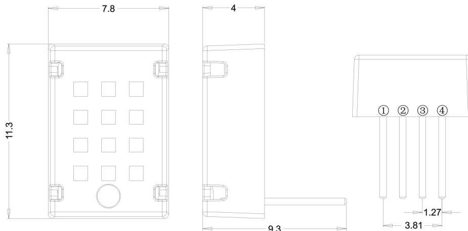
图1 AM2322 外形尺寸
