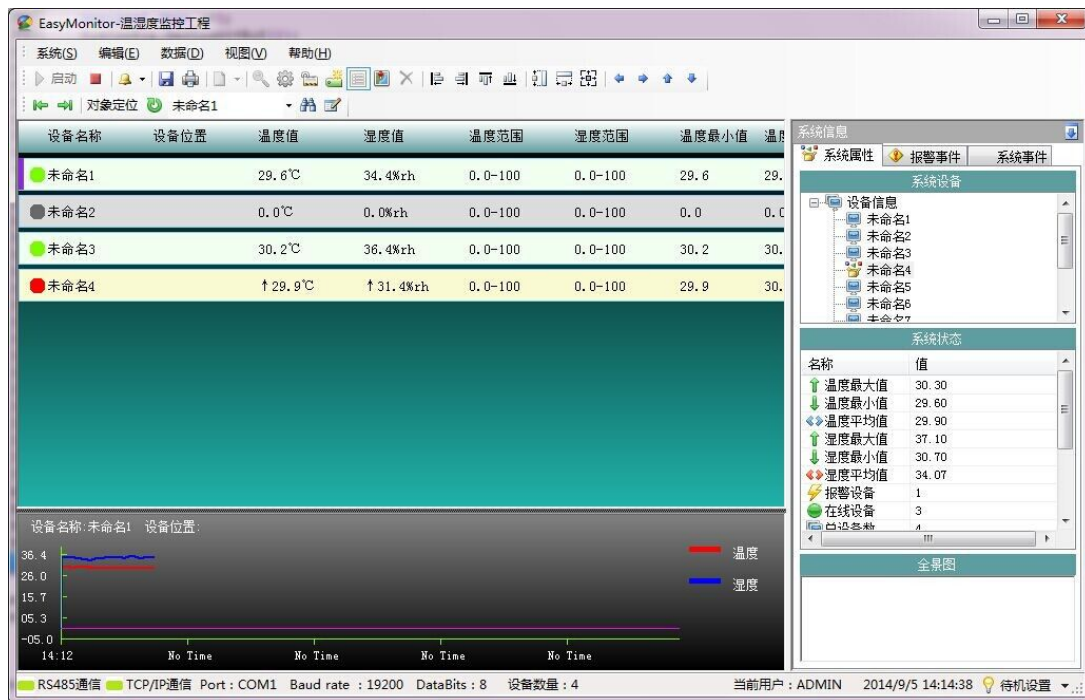
图 5 GSP885 变送器 485 监控软件
