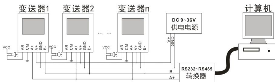
图 3 485 典型应用
