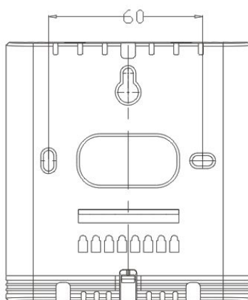
图 2 固定孔
