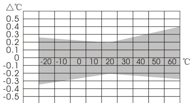
图10 -40~80°C 范围内对应的温度误差
