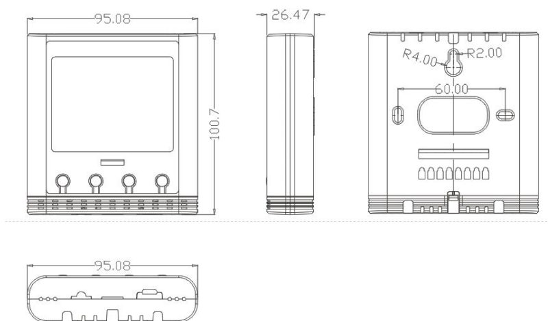
图 1 产品尺寸图（单位：mm）
