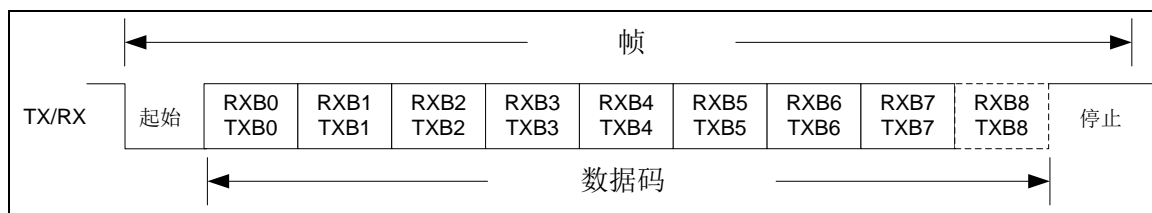
图 6-8 UART 数据格式示意图
