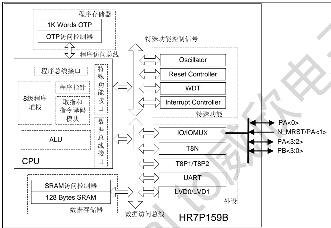
图 1-1 HR7P159B 结构框图
