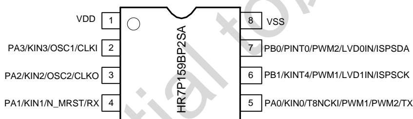
图 1-3 HR7P159B (SOP8) 顶视图
