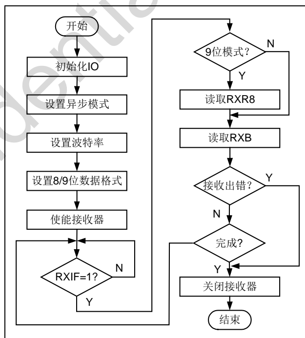
图 6-11 UART 接收器操作流程
