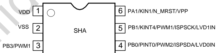
图 1-4 HR7P159B(SHA) (SOT23-6) 顶视图
