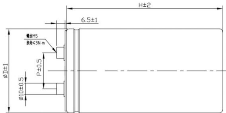
1000F~2400F螺栓系列产品尺寸规格
