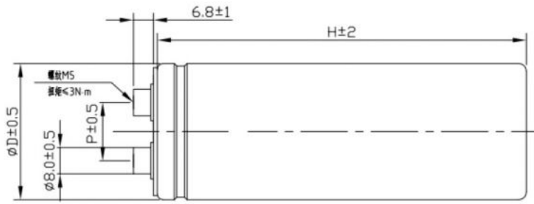
650F~800F螺栓系列产品尺寸规格
