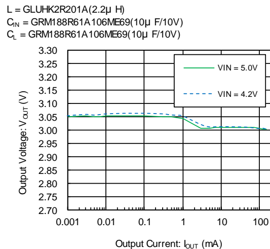
XC9276( V_{OUT}=3.0V )
