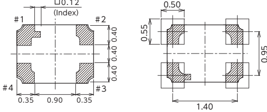
■ 焊盘图形 (参考) <Top View>
