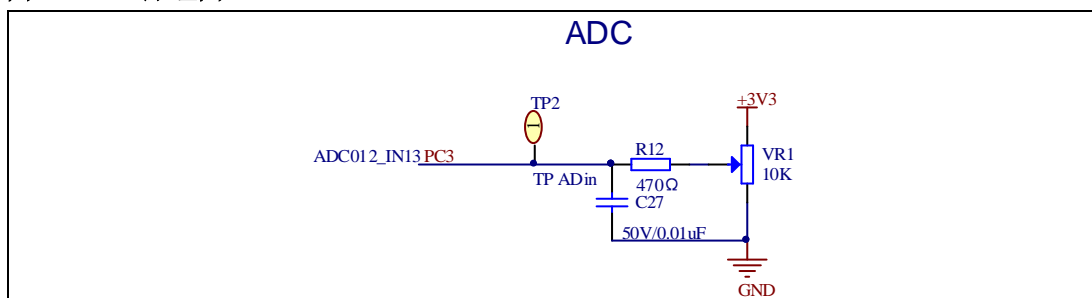
图4-5. ADC原理图
