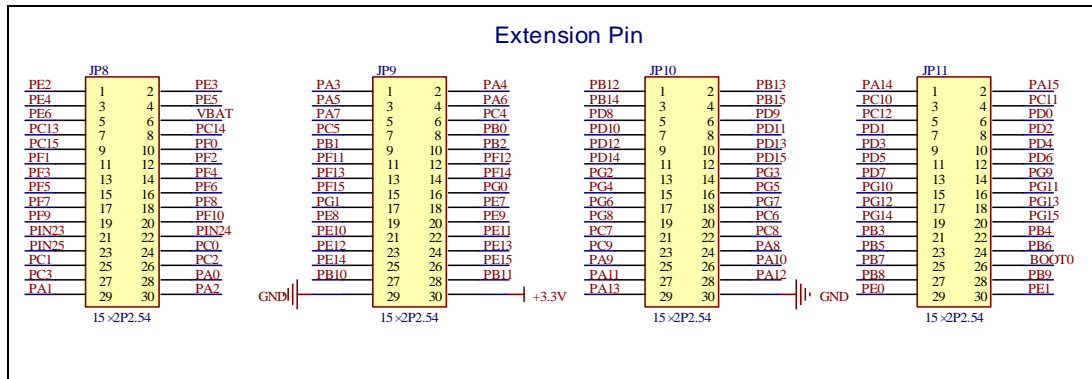
图4-16. Extension原理图
