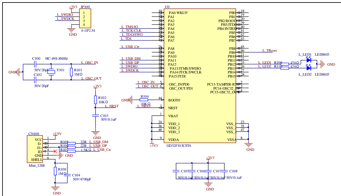
图4-17. GD-Link原理图
