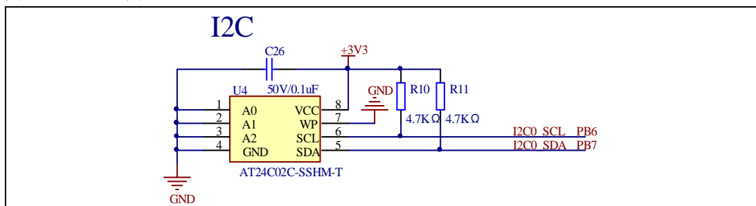
图4-9. I2C原理图
