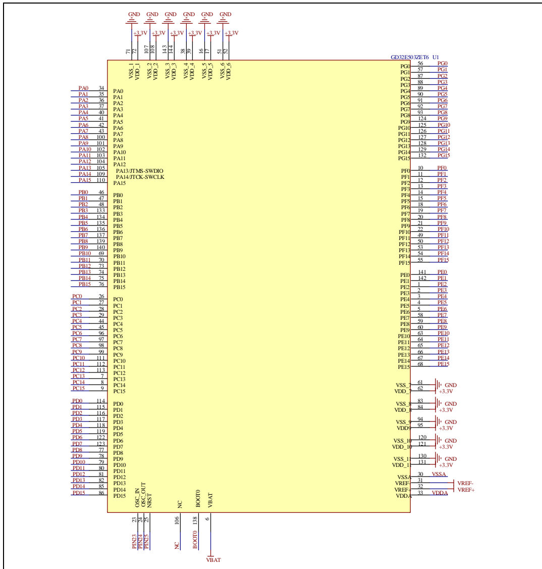
图4-18. MCU原理图
