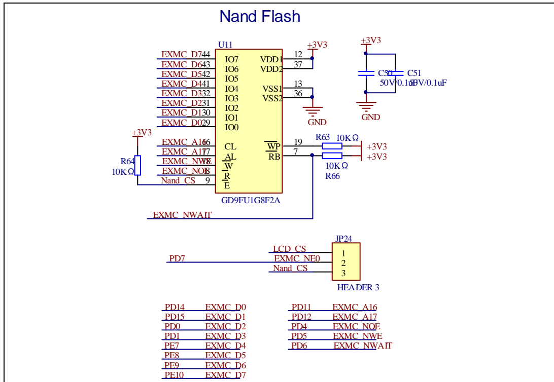
图4-11. NAND原理图
