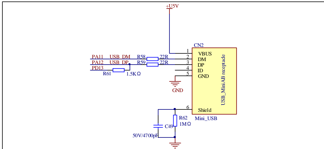
图4-14. USB原理图
