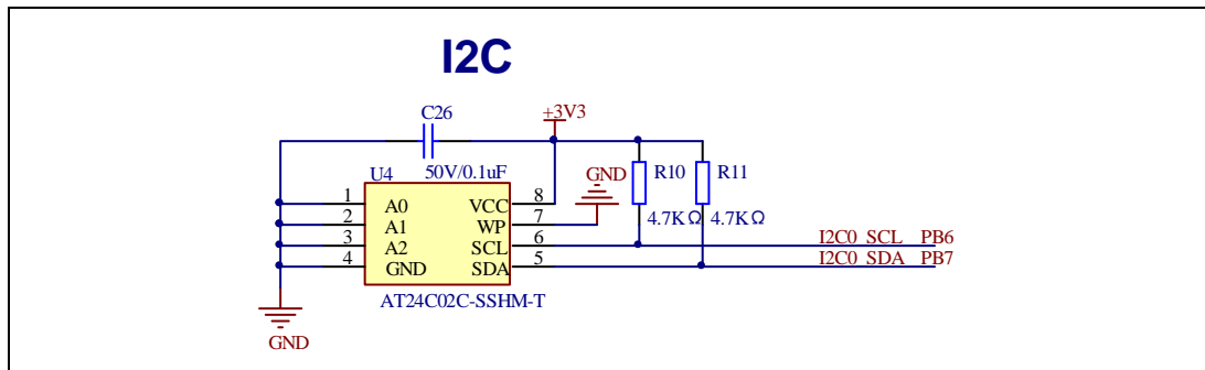
图4-8. I2C原理图
