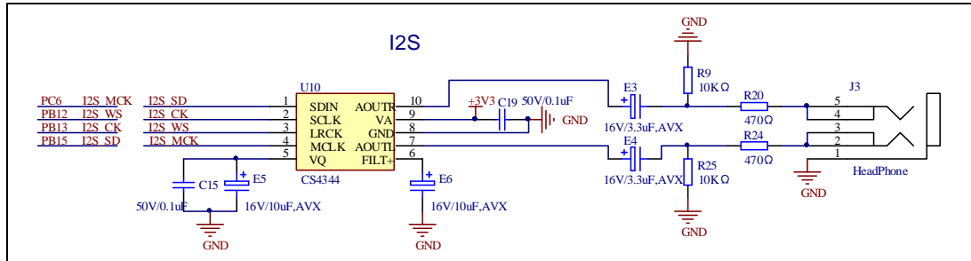
图4-9. I2S原理图
