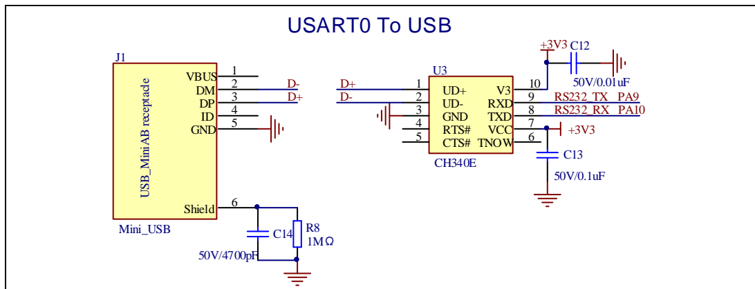
图4-7. USART原理图
