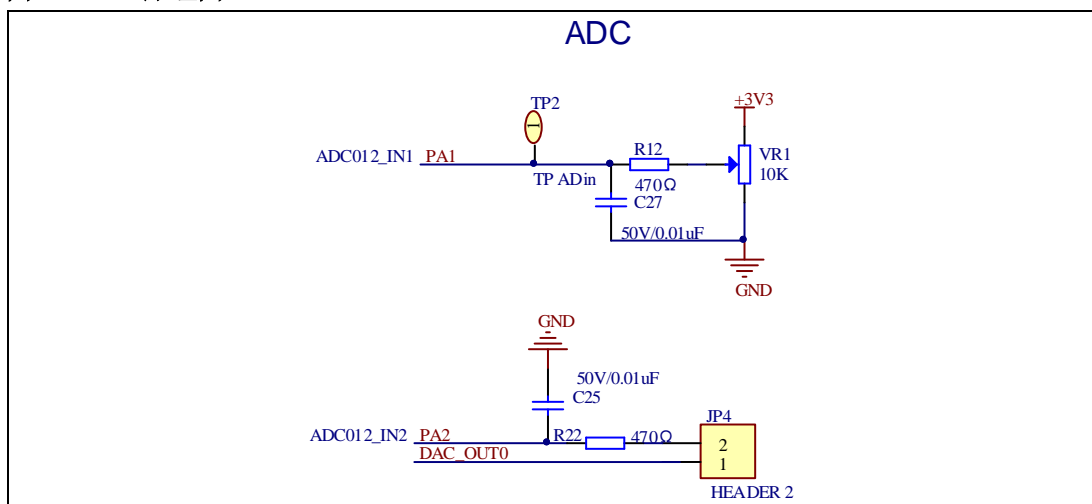
图4-5. ADC原理图
