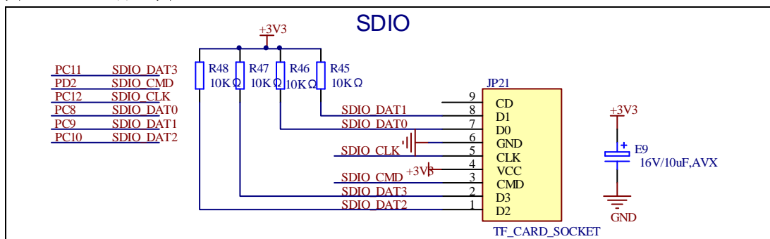
图4-13. SDIO原理图
