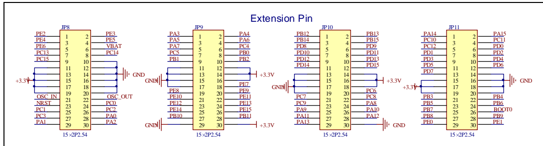
图4-15. Extension原理图
