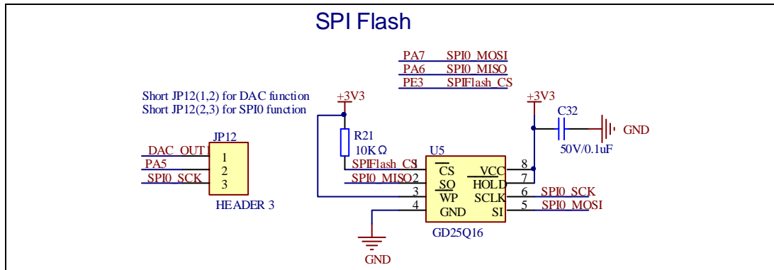
图4-10. SPI原理图
