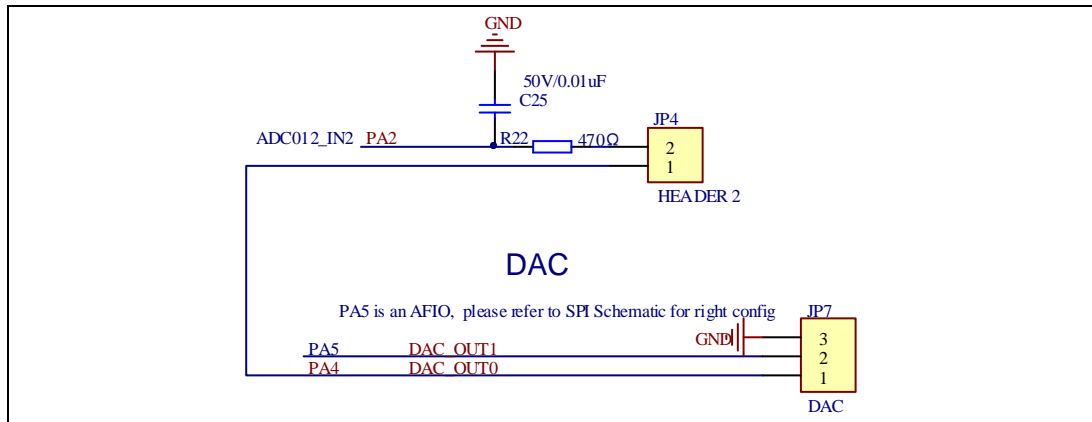
图4-6. DAC原理图
