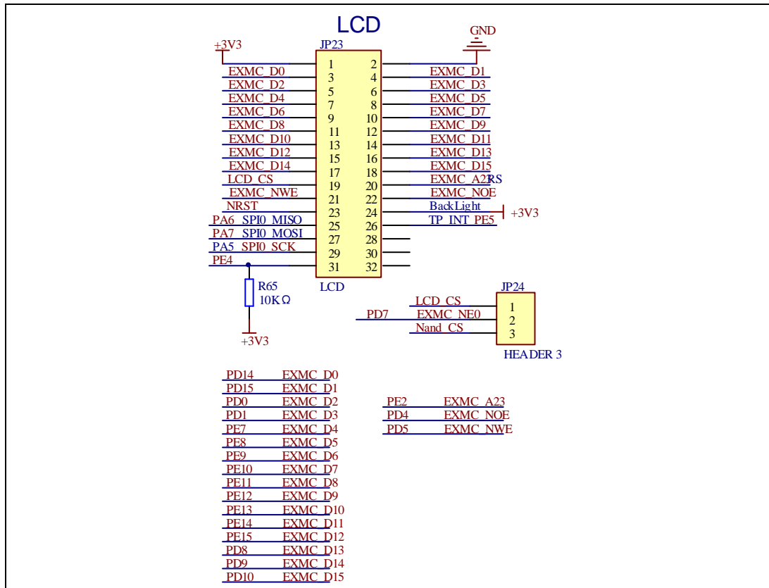
图4-12. LCD原理图
