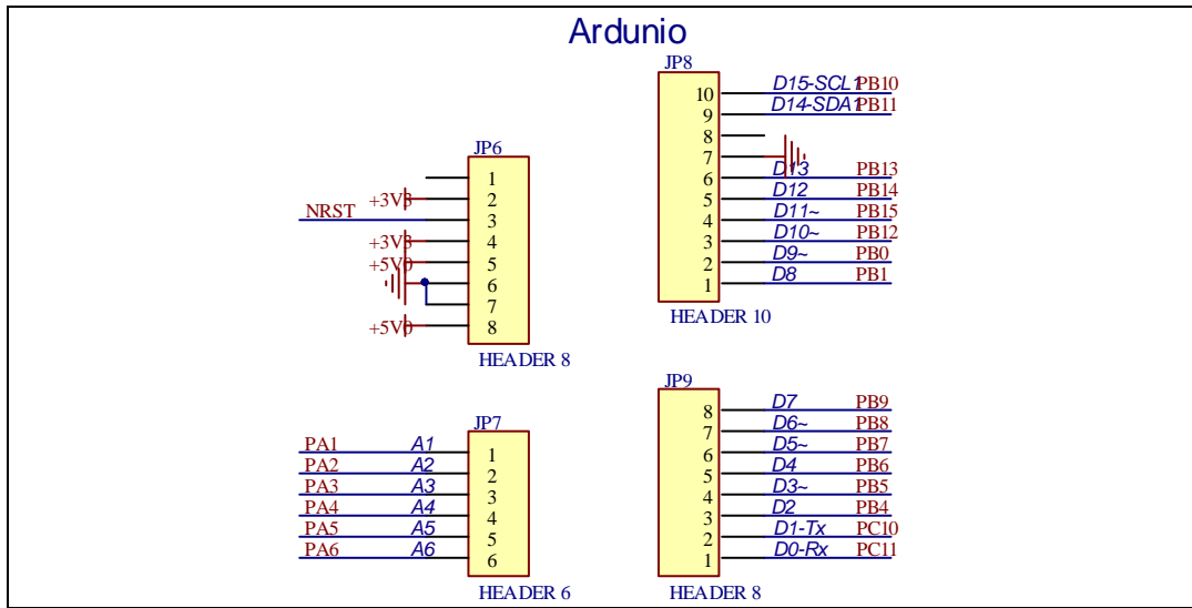
图4-9. Arduino原理图
