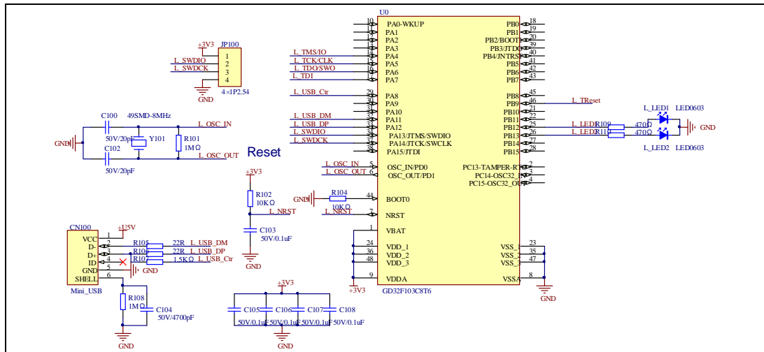
图4-8. GD-Link原理图
