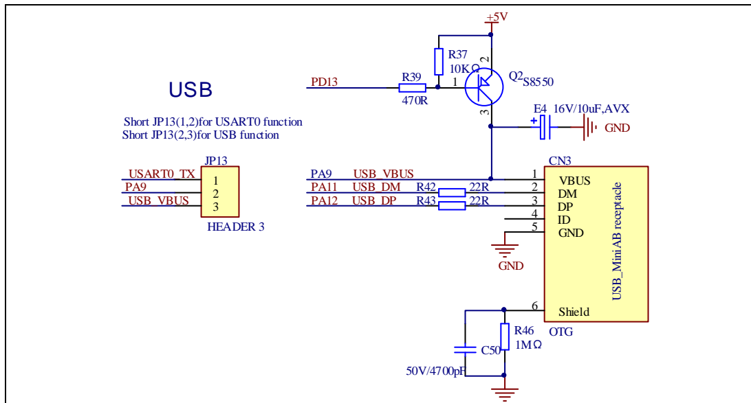
图4-15. USB原理图
