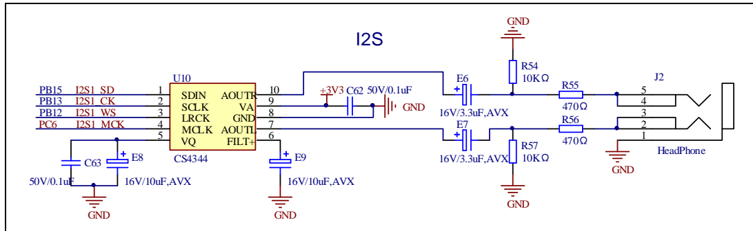
图4-10. I2S原理图
