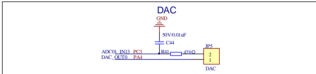
图4-6. DAC原理图
