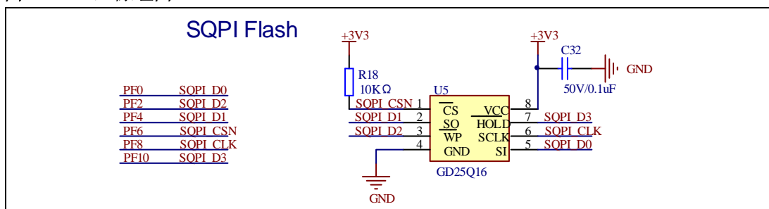
图4-11. SQPI原理图
