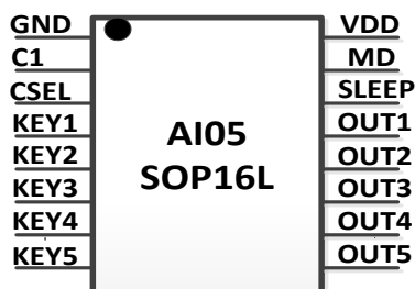
芯片引脚图
