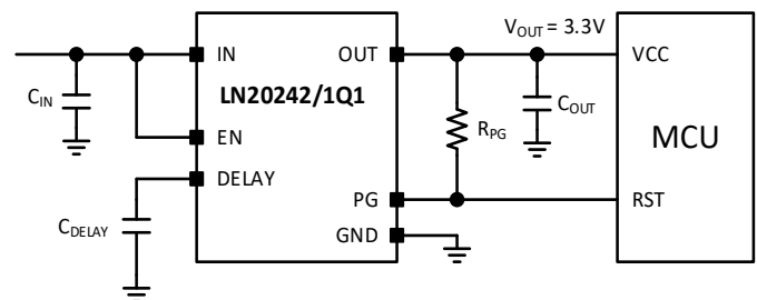
典型 MCU 应用图
