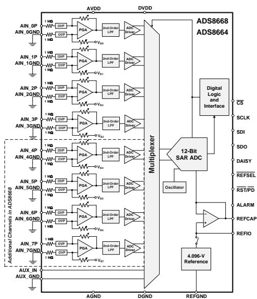
框图
