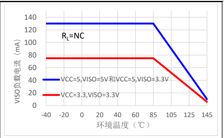
图 7.10-14 V ISO 最大负载可用电流随器件环境温度的变化 A 和 B 之间 R L = NC, CA-IS2092x 无发送和接收数据
