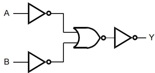
图 3 逻辑框图
