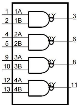
图 1 逻辑符号
