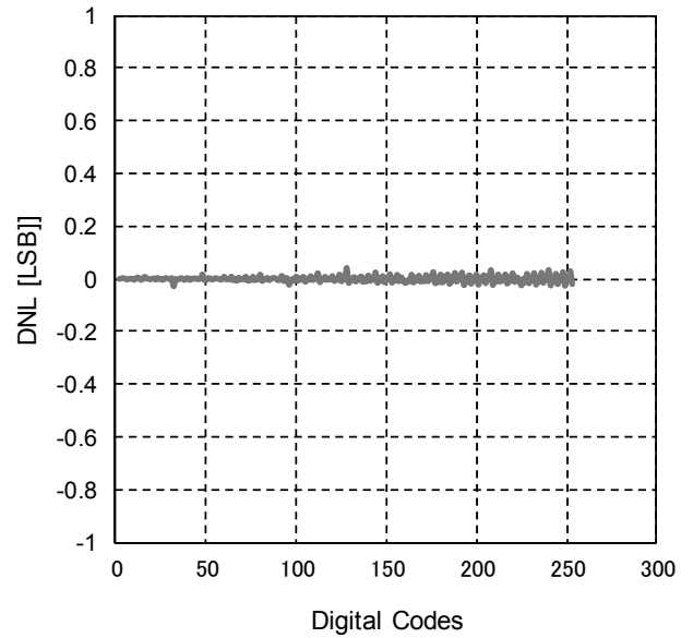
Fig.40 HAVDD DNL
